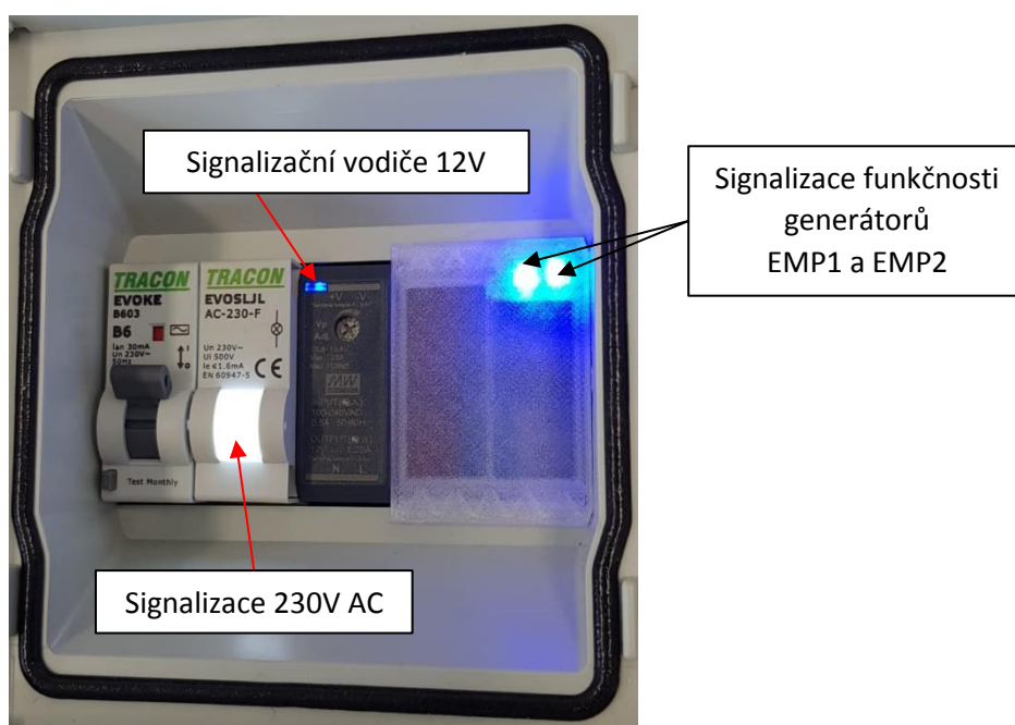
Obrázek SEQ Obrázek \* ARABIC 2 Rozvaděč, světelné kontrolky
